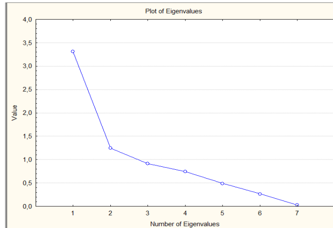
Рисунок 5. Графік кам'янистій осипи
