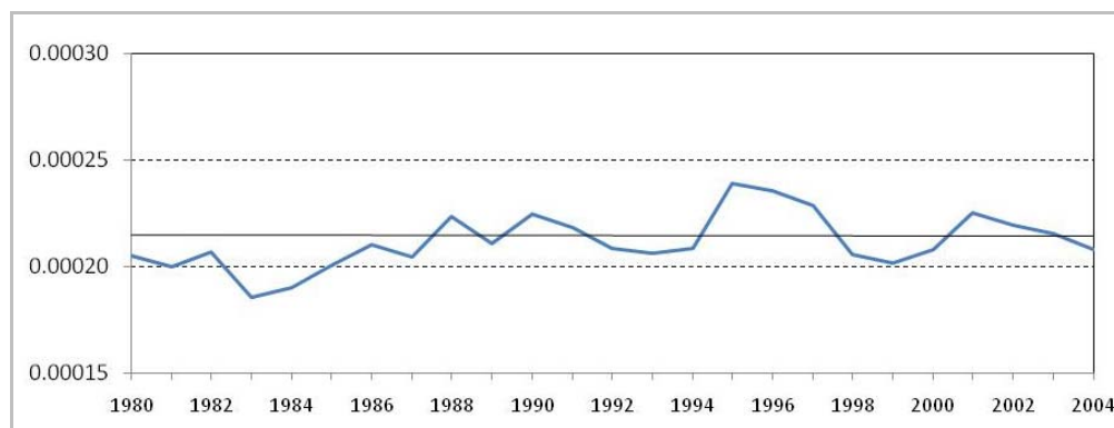
Fig. 11. CO 2 emissions (1980-2004)
