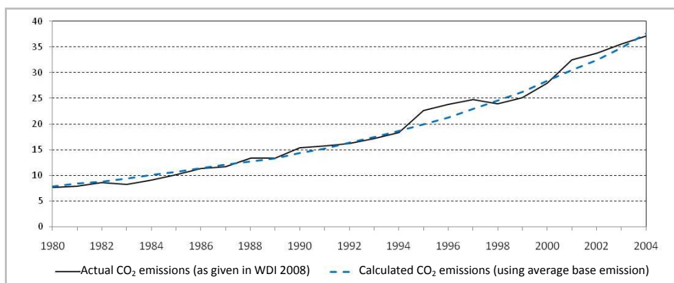
Fig. 11. CO 2 emissions (1980-2004)
